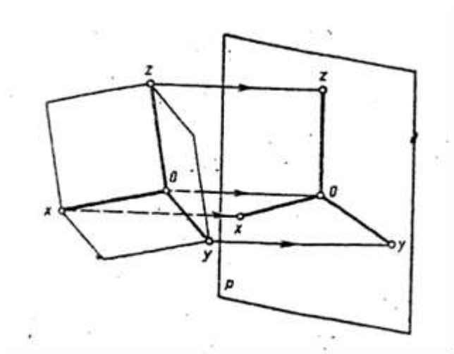
Рис.23 Направление проецирующих лучей в аксонометрии
