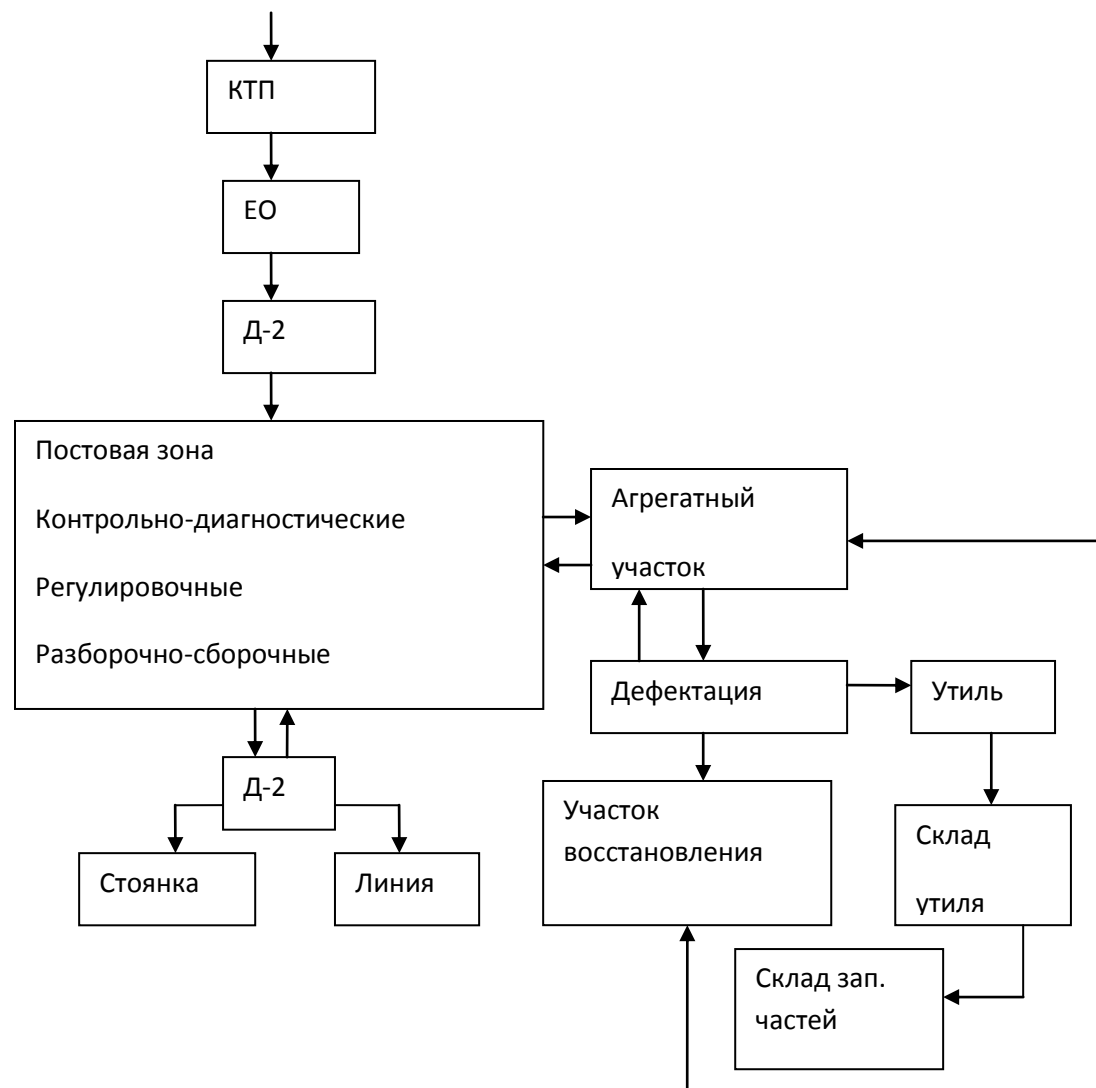
Рисунок 4 Технологический процесс зоны ТР
