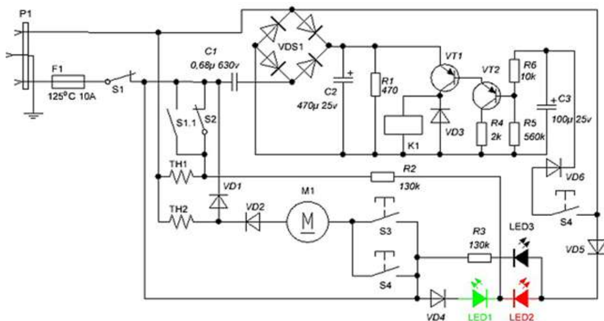
Рис. 10 Принципиальная схема термopота
