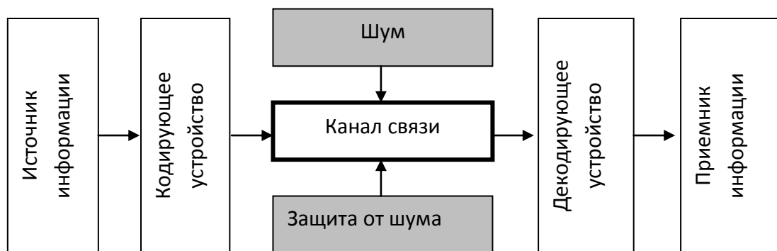
Рисунок 2 – Схема процесса передачи информации по техническим каналам связи
