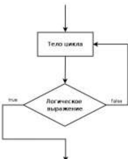
Цикл repeat
