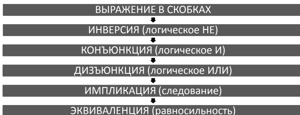
Рисунок 3 – Приоритет логических операций
