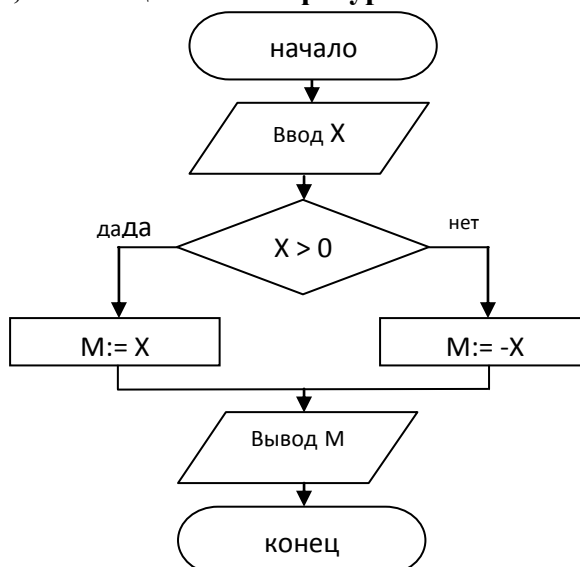
Рисунок 1 – Разветвляющийся алгоритм
