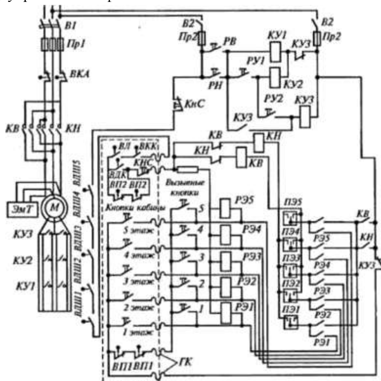
Рисунок 1 - Электрическая схема пассажирского лифта
