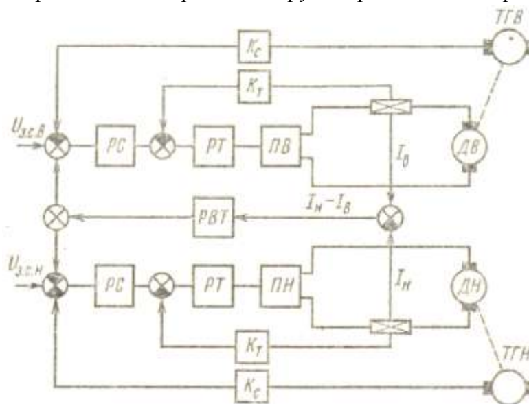
Рисунок 1 -Схема выравнивания токов с сепаратным управлением
