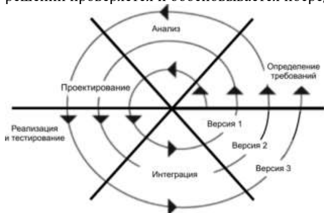
Рис. 3. Спиральная модель жц системы.
