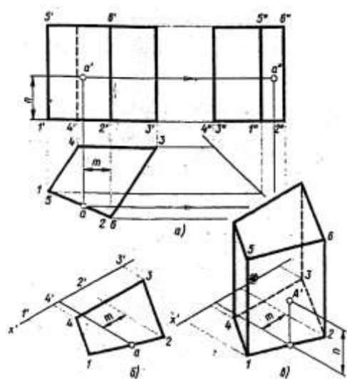
Рис.6 Проекция призмы
