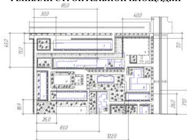
ГЕНПЛАН СТРОИТЕЛЬНОЙ ПЛОЩАДКИ
