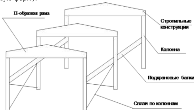
Рис. 3.1. Каркас здания
