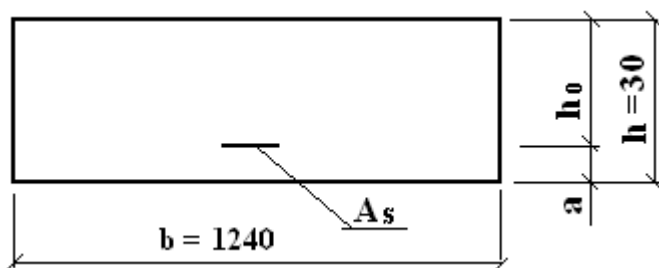
Рисунок 13 - Расчетное сечение полки
