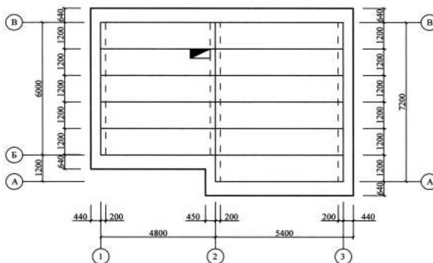
Рис. 3.5. План безбалочного перекрытия
