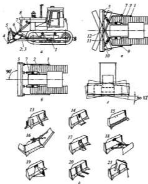
Рисунок 2. Бульдозер: а – вид сбоку; б – вид в плане на бульдозер с неповоротным отвалом; в – то же, с поворотным отвалом; г – перекоос отвала; д – сменные рабочие органы.
