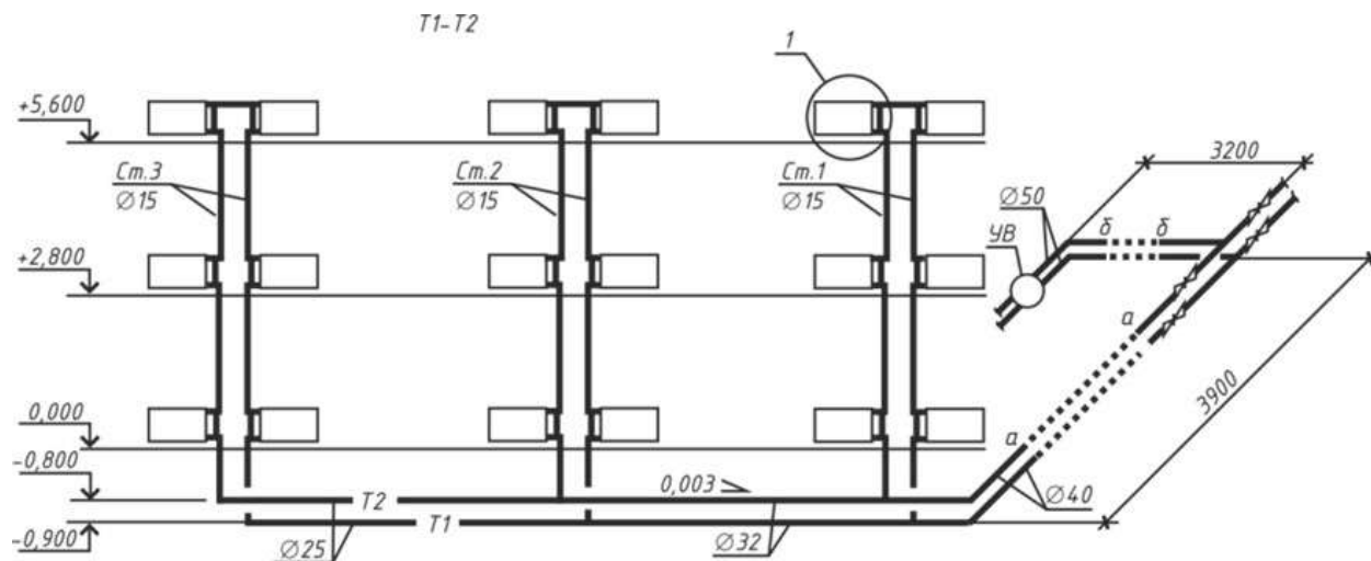
Рисунок 4. Фрагмент схемы системы отопления Т1, Т2
