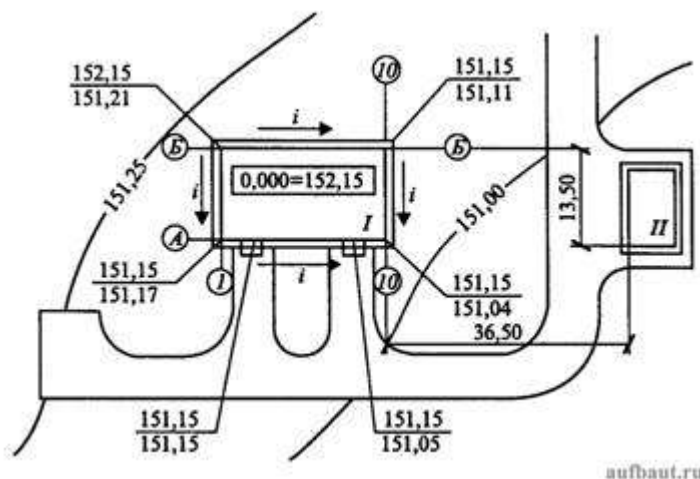
Рисунок 1. Пример выполнения вертикальной и горизонтальной привязок в учебной практической работе: I - проектируемое здание; II - существующее здание; i - направление стока поверхностных вод; A, B, 1, 10 - обозначения осей
