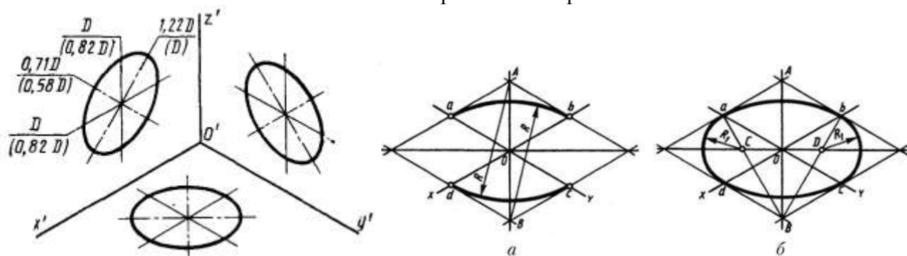
Рис.17 Аксонометрия окружности
