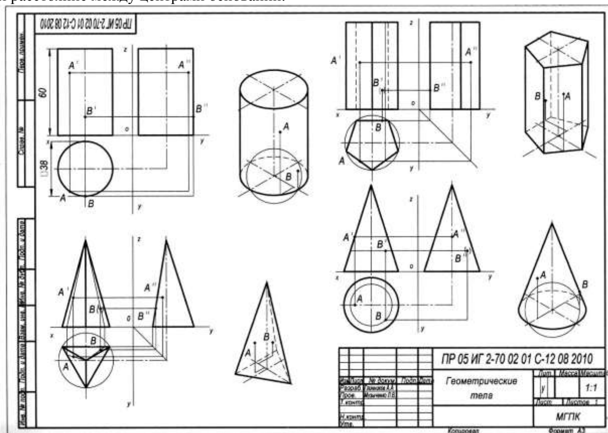
Рис.19 Пример оформления графической работы
