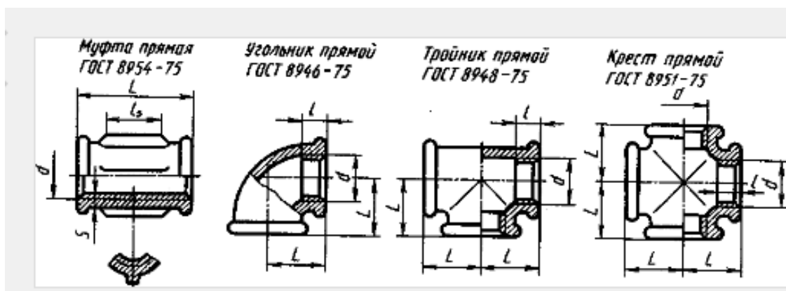
Рис. 70 Примеры фитингов
