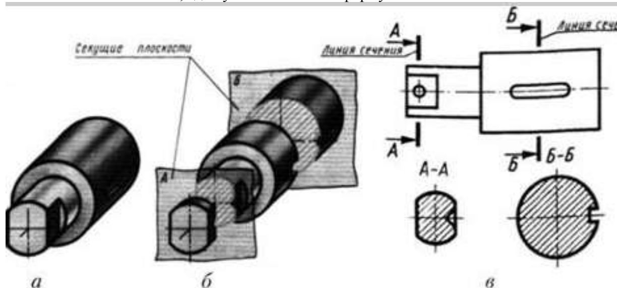
Рис. 50. Образование сечений
