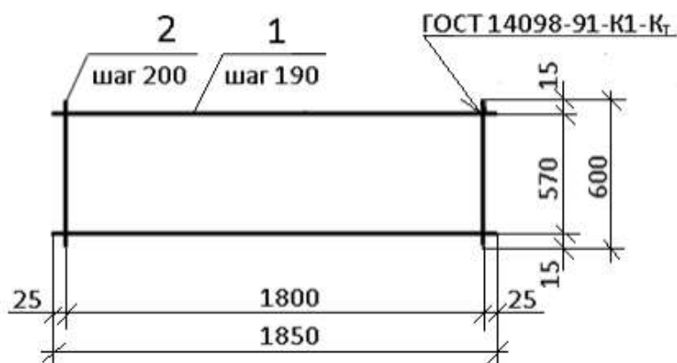
Рис. 93 Сборочный чертёж сетки
