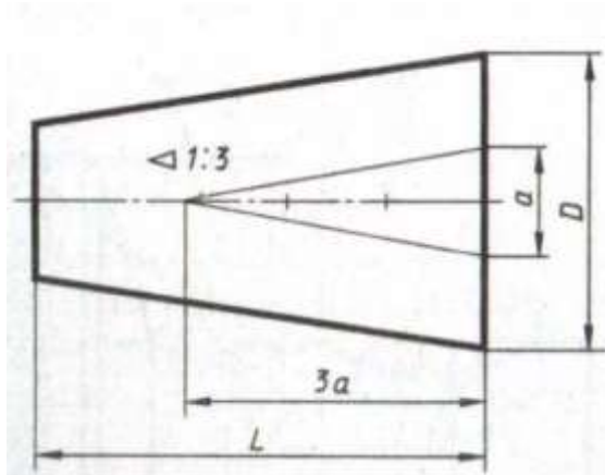
Рис.5 Конусность
