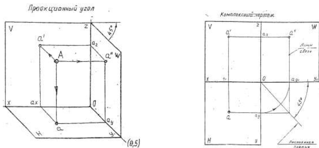
Рис.10 Проекция точки
