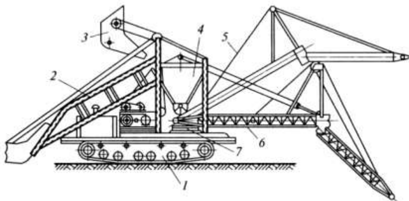
Рисунок 3. Самоходный бетоноукладчик.
