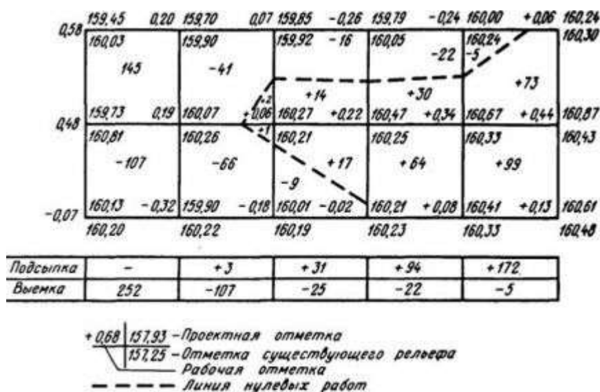
Рисунок 1. Подсчет объема земляных работ
