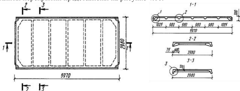
Рис. 4.10. Плиты перекрытий
