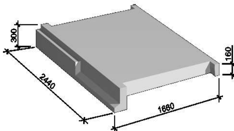
Рис. 9.22. Лесничная площадка железобетонная
