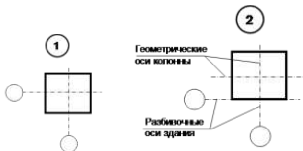
Рис. 3.4. Нулевая проекция
