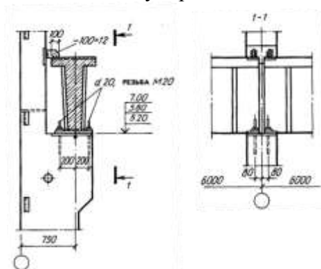
Рис. 4.5. Узел опирания подкрановой балки
