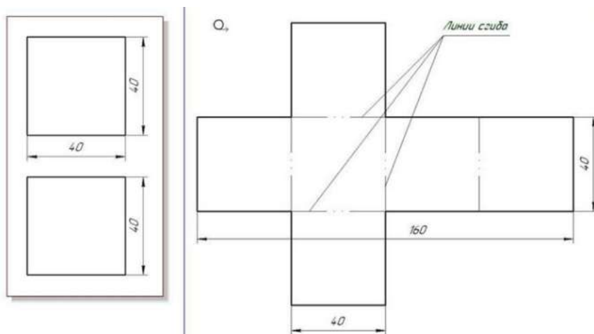
Геометрическое тело №2
