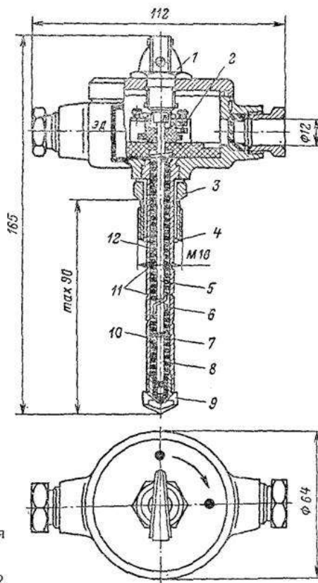
Рис. 1 - Датчик контроля температуры
