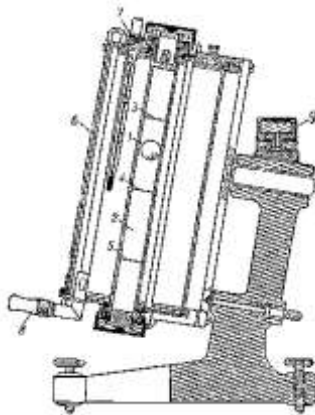
Рисунок 5 - Вискозиметр Гепплера со «скользящим» шариком: 1 — шарик; 2 — трубка с жидкостью; 3, 4, 5 — кольцевые метки на трубке; 6 — термостатирующая жидкостная баня; 7 — термометр; 8 — штуцер для присоединения прибора к термостату; 9 — уровень.
