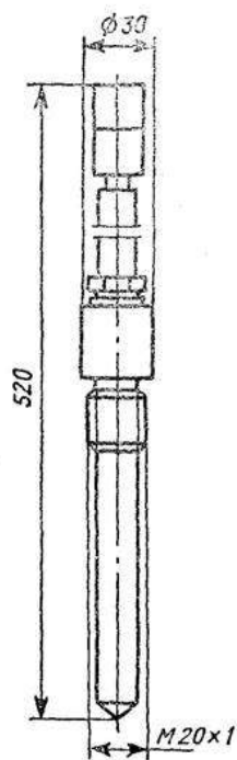
Рис. 36. Датчик контроля температуры ДКТ-1
