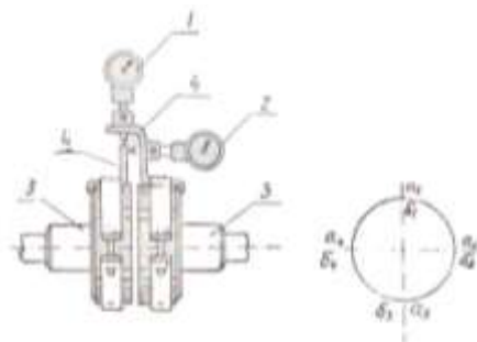
Схема измерения осей горизонтальной линией: 1 - индикатор для осей радиального биения; 2 - индикатор для осей торцевого биения; 3 - муфта; 4 - скоба
