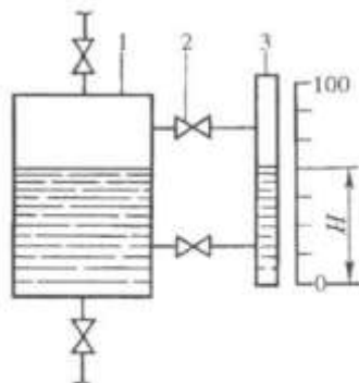
Рис. 1. Визуальный уровнемер.
