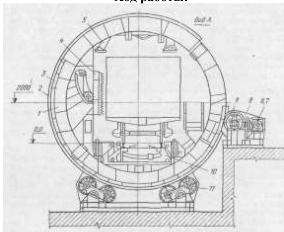
Рисунок 6 – Схема стационарного роторного вагоноопрокидывателя
