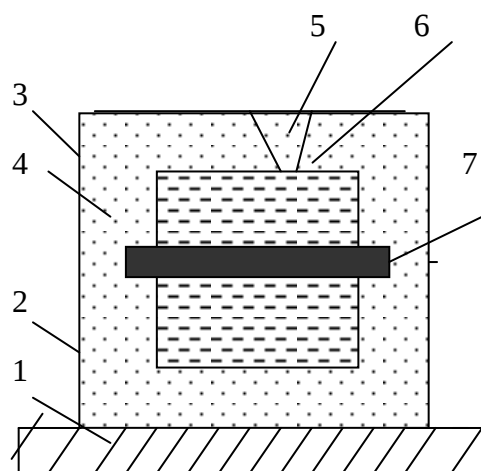
Рис. 1. Литейная форма
