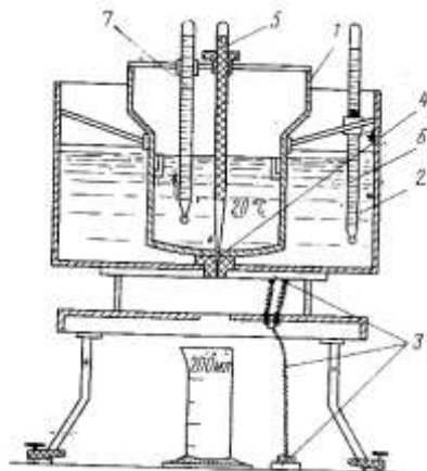
Рисунок 1 - Схема вискозиметра Энглера
