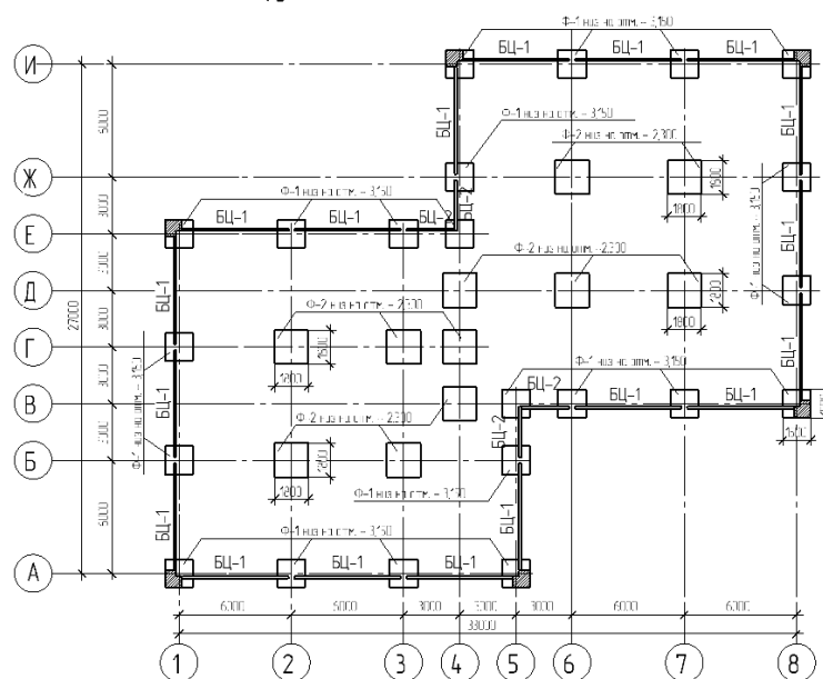
План фундаментов
