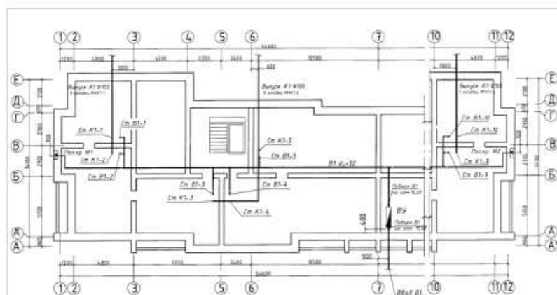
Рис. 2. План технического подполья
