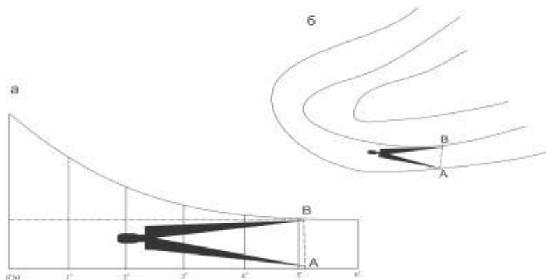
Рис. 15. схема определения крутизны ската по графику заложений
