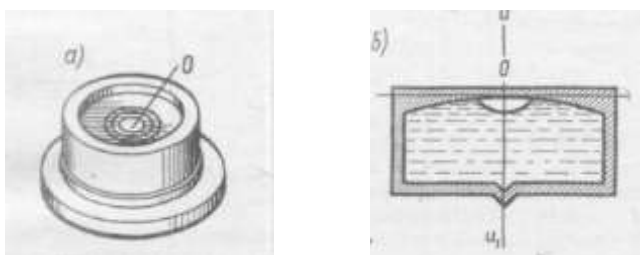
Рисунок 6. Круглый уровень:
