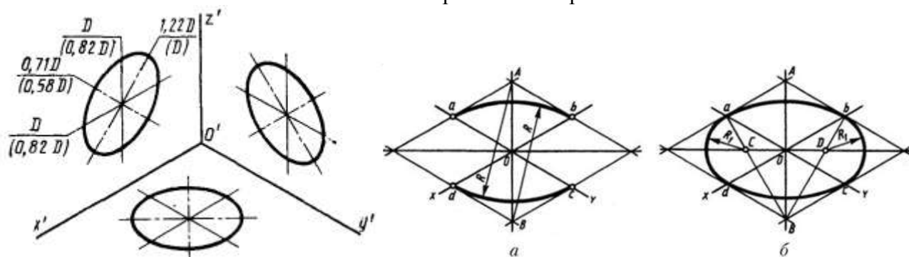
Рис.17 Аксонометрия окружности
