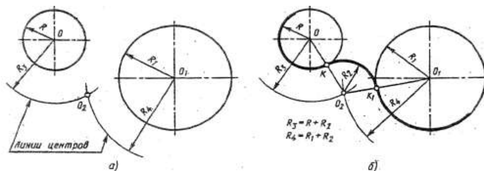
Рис.8 Внешнее касание
