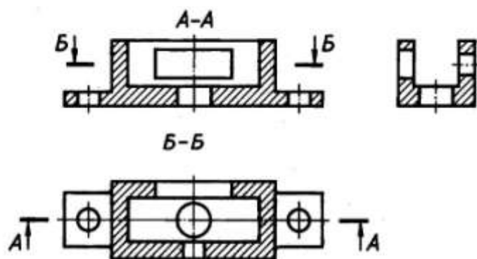
Рис. 56. Обозначение разрез
