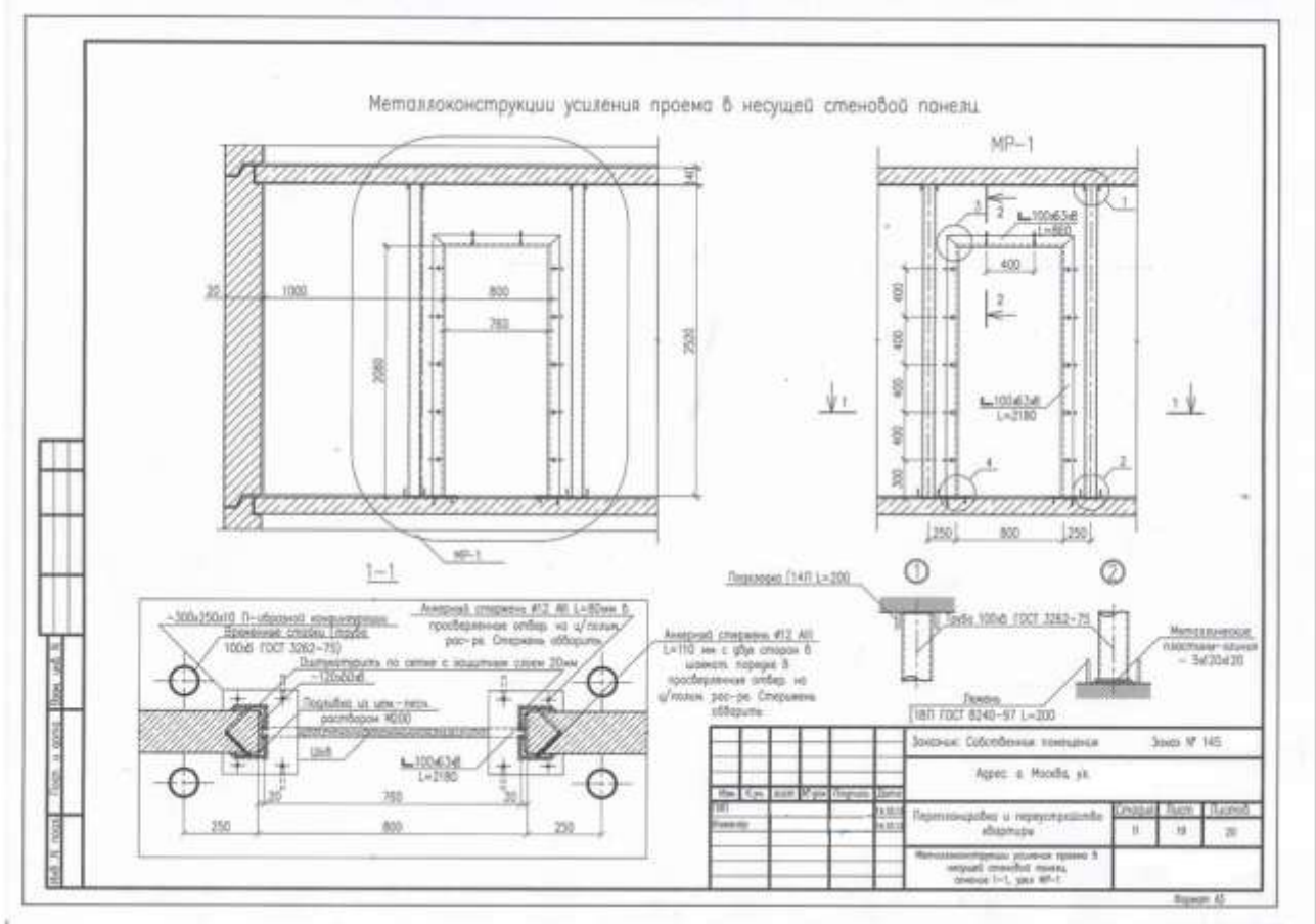
Рисунок 8.1 – Пример оформления чертежа усиления проёма
