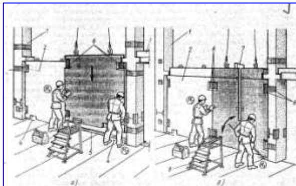
Рисунок. Установка безригельной панели жёсткости:
