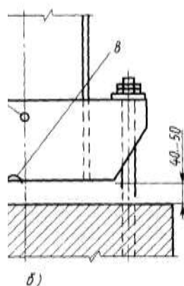
Рисунок 2.1 Схемы установки стальных колонн на фундаменты:
