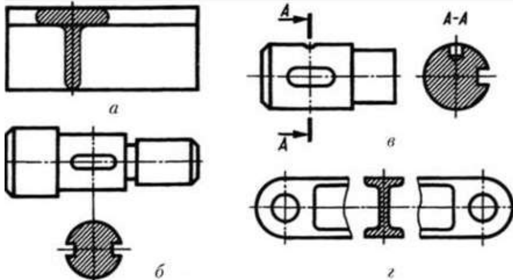
Рис. 51 Расположение сечений
