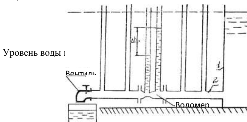
Рисунок 1 - Схема установки
