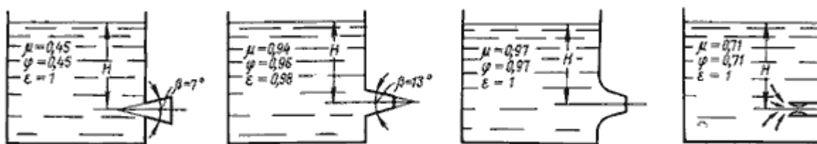
Рисунок 4- Истечение жидкости через насадки
