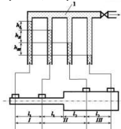
Рисунок -.1. Измерение разности напоров на местном сопротивлении. 1-блок дифференциальных пьезометров; l_1, l_2 –длины участков I и II; l_3, l_4 –длины участка III непосредственно перед и после внезапного расширения; h_1, h_2, h_3 , - потери напоров на участках I, II, III.
