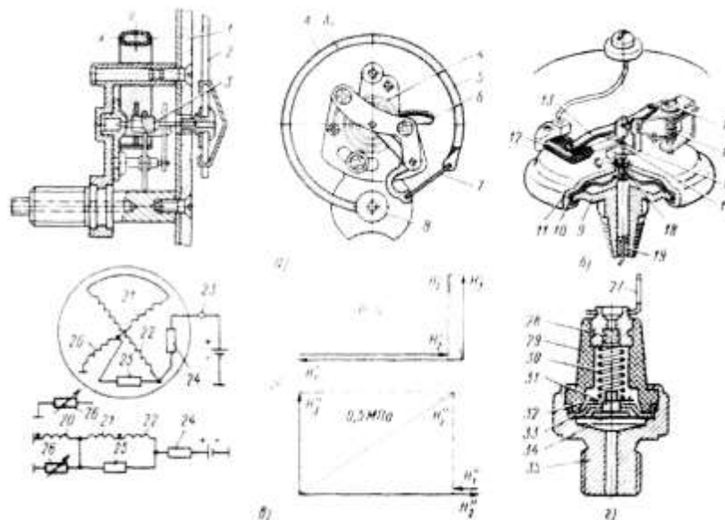
Рисунок 2. Указатель давления: а) механизм указателя с трубчатой пружиной;
