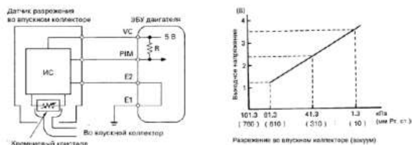
Рисунок 7: а - схема включения датчика абсолютного давления коллектора; б - характеристика датчика МАР
