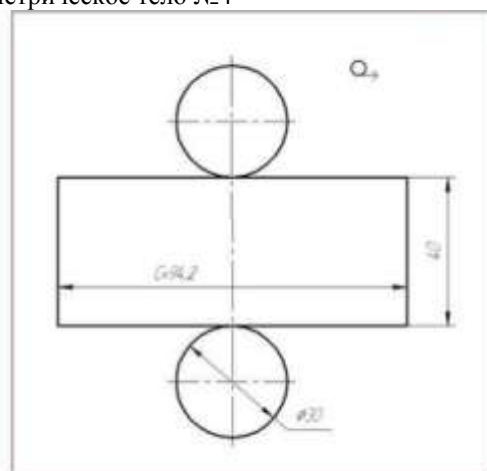
Геометрическое тело №4
