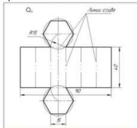
Геометрическое тело №4
