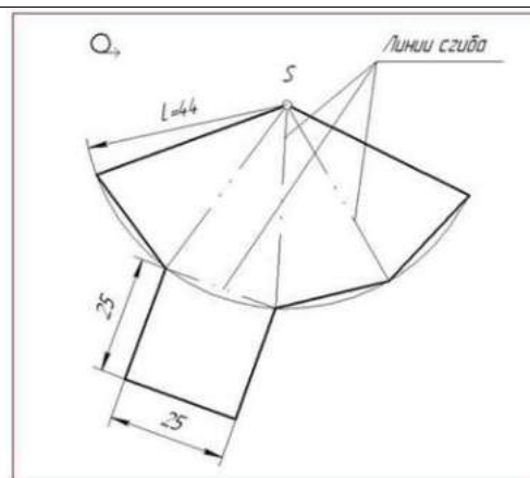
Геометрическое тело №4
