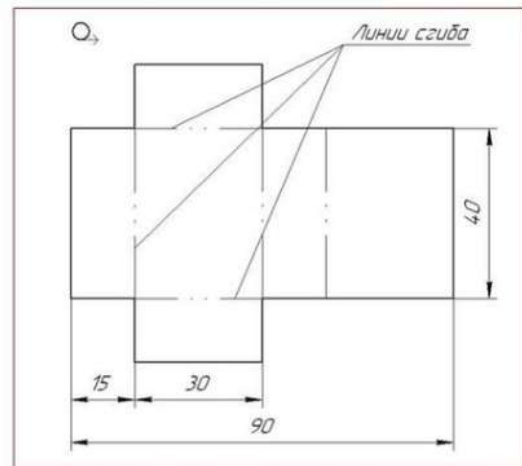
Геометрическое тело №3
