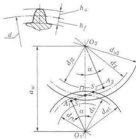
Рис. 18.1. Геометрия цилиндрической передачи: P — полюс зацепления; A_1A_2 — линия зацепления; S_1S_2 — длина активной линии зацепления; \alpha — угол зацепления; a_w — межосевое расстояние; d_1, d_2 — диаметры делительных окружностей; h_a, h_f — высота головки и ножки зуба соответственно; d_{f1}, d_{f2} — диаметры окружностей впадин; d_{a1}, d_{a2} — диаметры окружностей выступов
