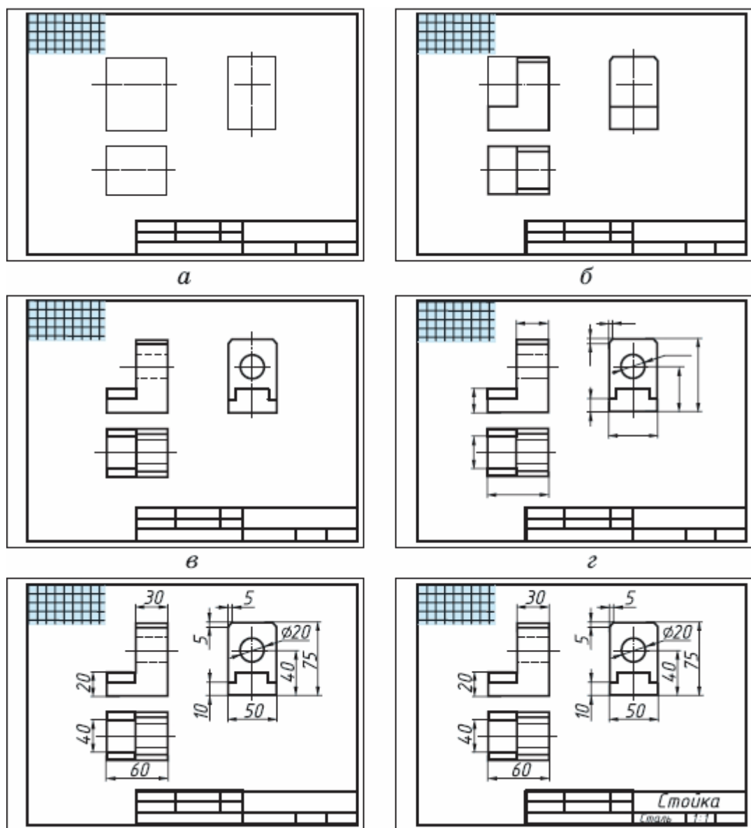
Рис.44 Последовательность выполнения эскиза детали
