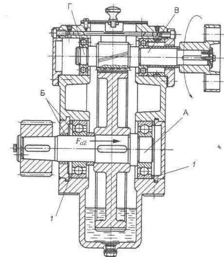
Деталь 15.2
