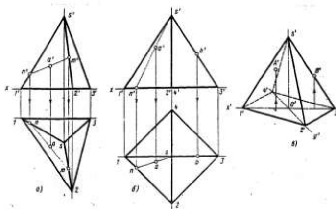
Рис.7 Проекция пирамиды
