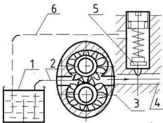
Рис. 1. Схема шестерённого насоса: 1 - масляный резервуар; 2, 6 - трубопровод; 3 - замкнутая камера насоса; 4 - нагнетательный трубопровод; 5-предохранительный клапан
