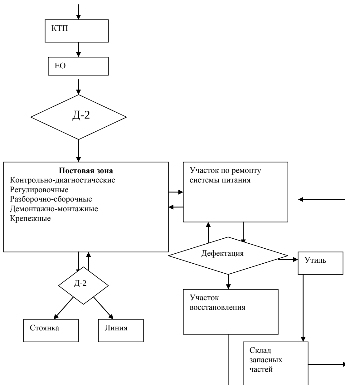
Рисунок 3 – Схема технологического процесса ТР АТП
