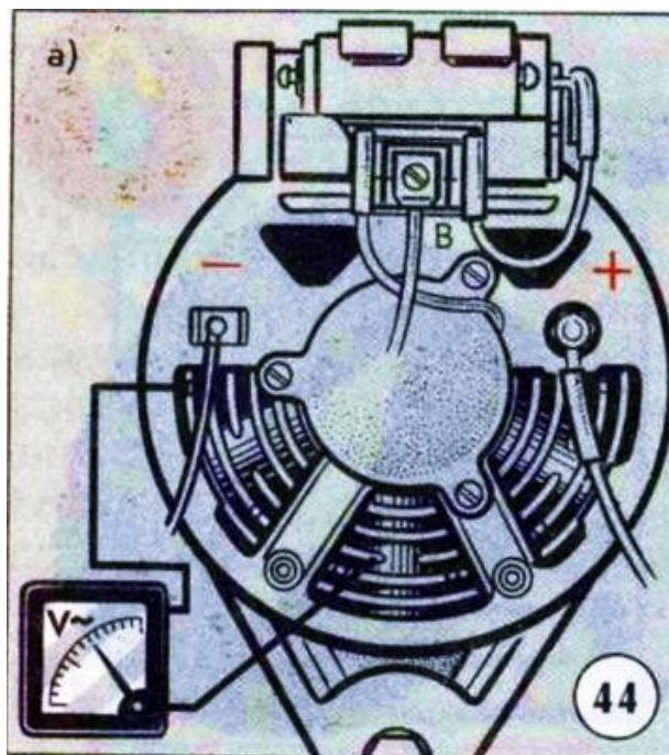
Рисунок 3. Проверка на автомобиле обмотки статора генератора с выпрямительными блоками БПВ (а) и ВБГ (б)
