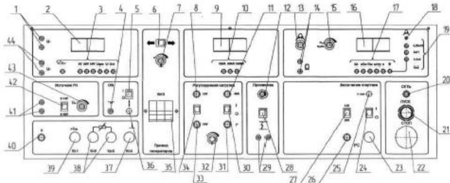
Рисунок 5. Панель управления:
