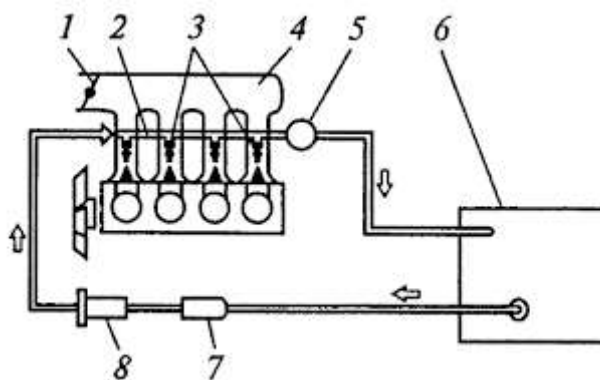
Рис. 4 Схема системы питания двигателя
