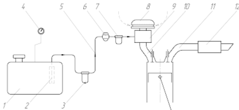
Рис. 1. Схема системы питания карбюраторного двигателя
