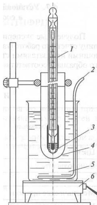
Рис. 7. Прибор для определения температуры каплепадения смазок:
