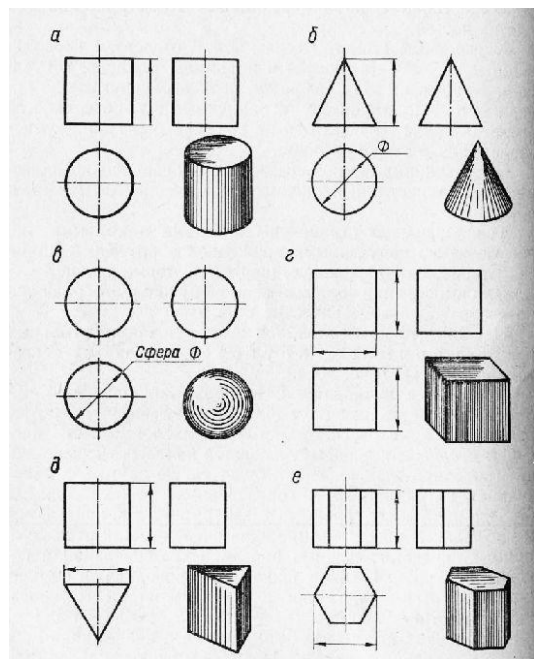
Рис.10 Проекции геометрических тел призмы
