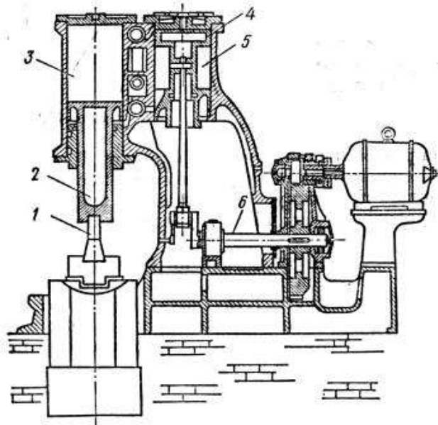
Рис. 6 Паровоздушный молот
