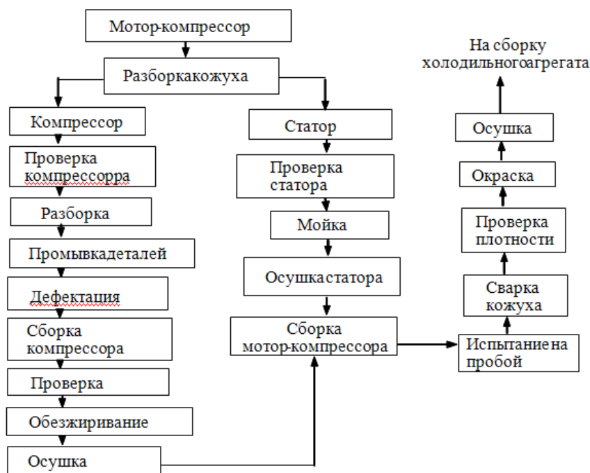
Рис. 2 Схема ремонта мотор-компрессора
