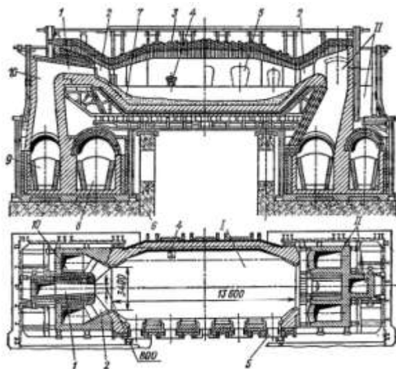
Рис. 2. Мартеновская печь:
