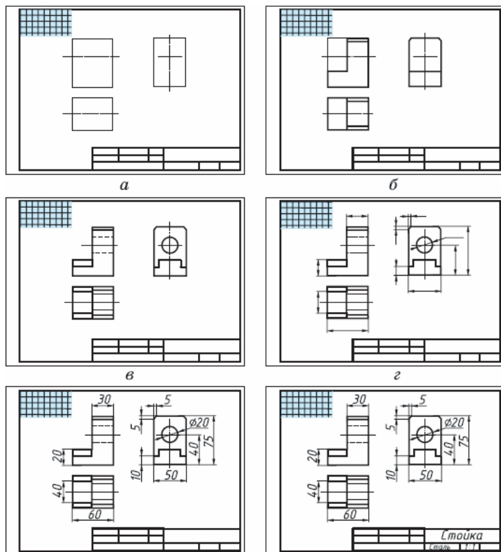
Рис.44 Последовательность выполнения эскиза детали
