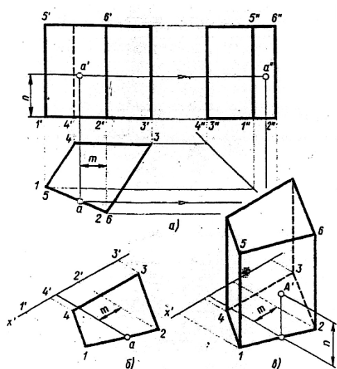
Рис.6 Проекция призмы
