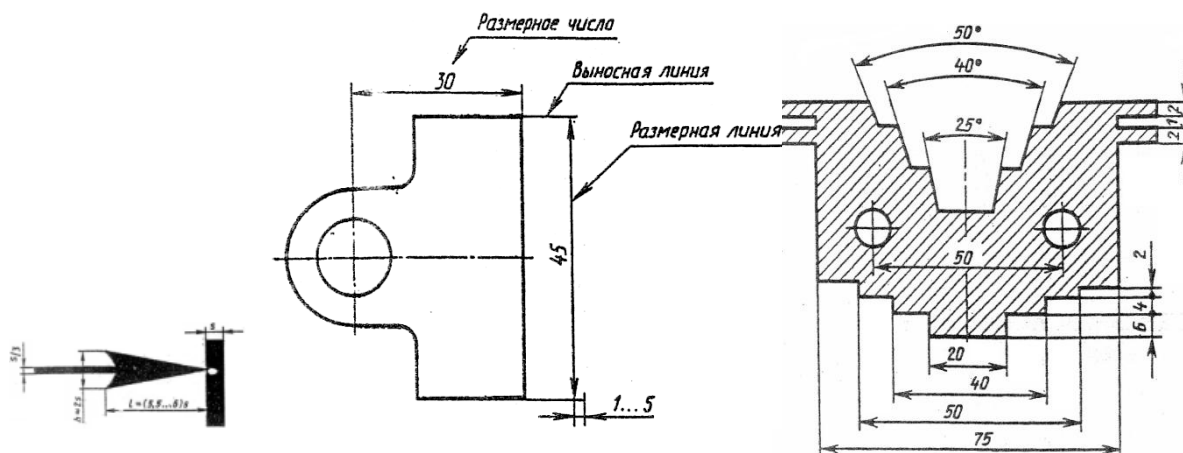
Рис.3 Нанесение размеров
