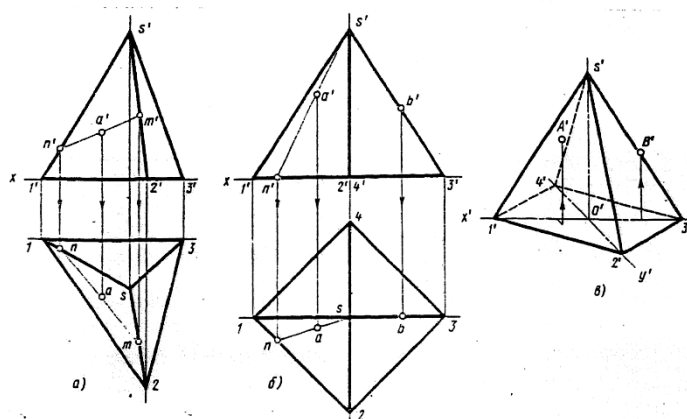
Рис.7 Проекция пирамиды
