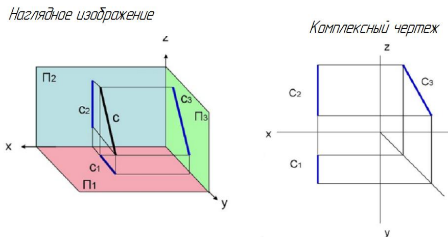
Рис.5 Проекции прямой
