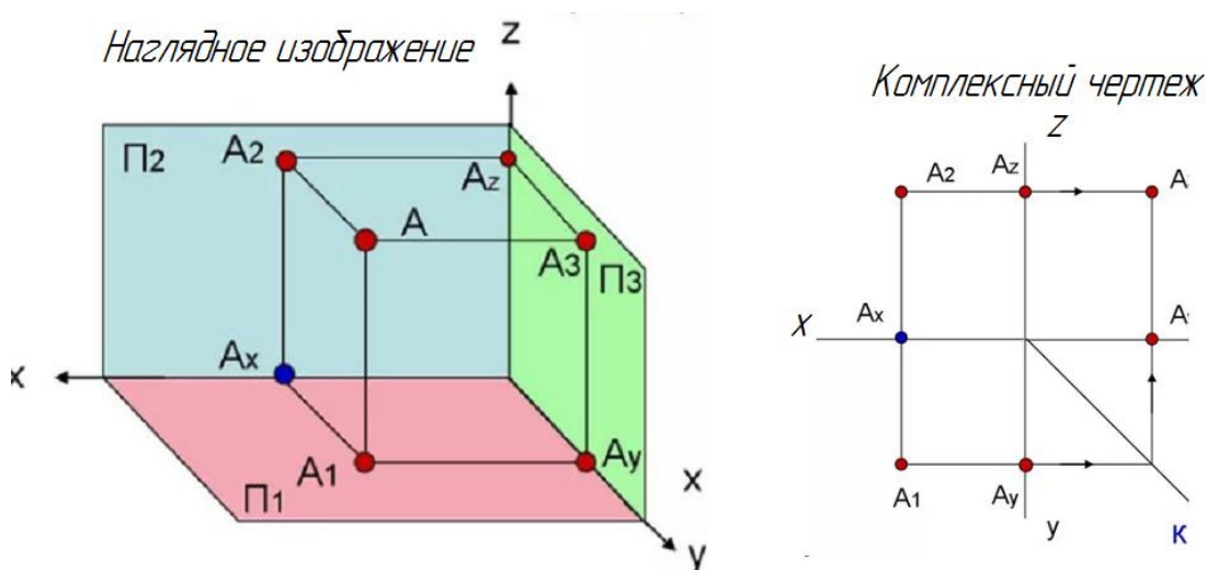
Рис.4 Проекция точки
