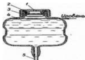
Питательный бачёк главного тормозного
