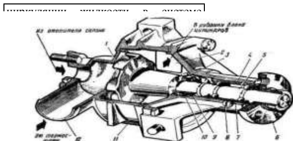
Рис. 7. Центробежный водяной насос двигателя автомобиля ВАЗ-2106:
