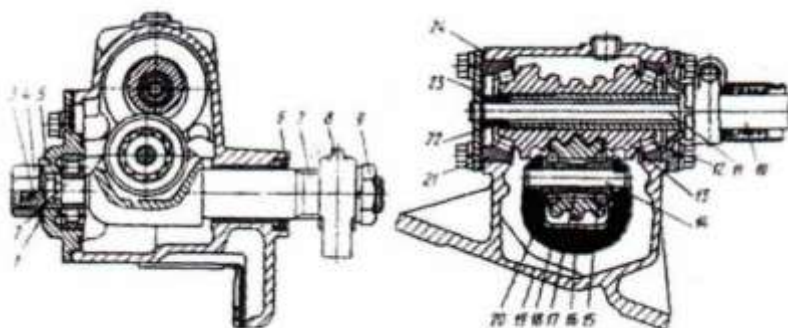
Устройство рулевого механизма
