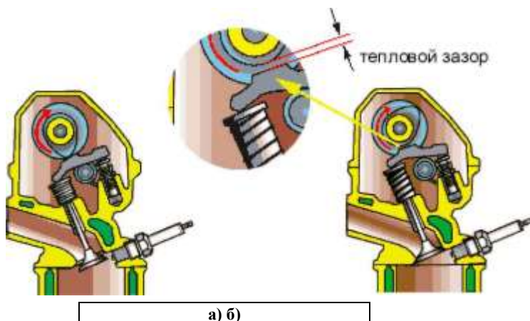
Рис. 12 Схема взаимодействия деталей газораспределительного механизма а) б)
