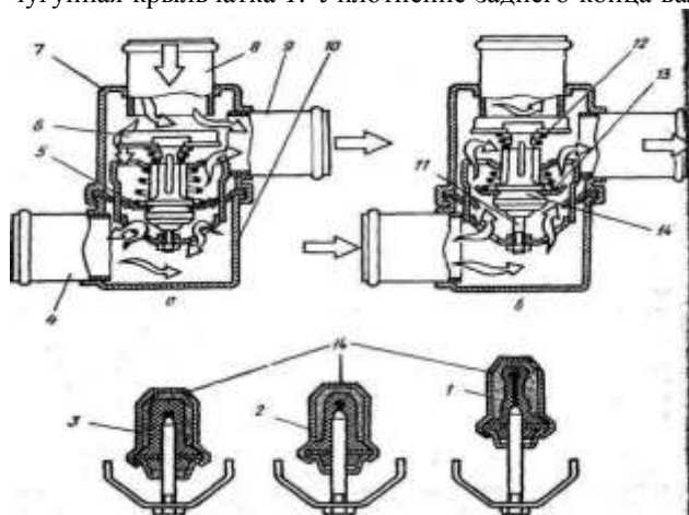
Рис. 9. Устройство и работа термостата
