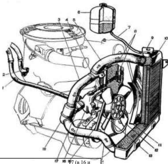
Рис. 5. Система охлаждения двигателя автомобиля ВАЗ-2106: 1—патрубок отвода жидкости из отопителя; 2—патрубок подвода горячей жидкости из головки блока цилиндров в отопитель; 3 — шланг перепускного патрубка термостата; 4 —
