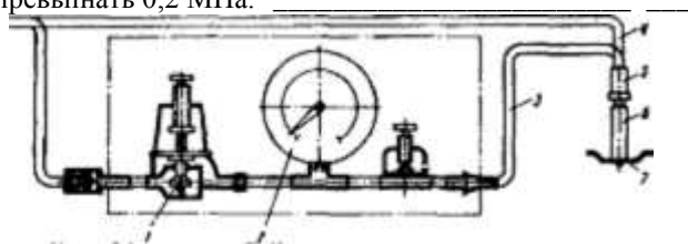
Прибор К-69М
