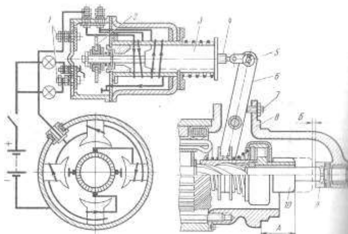
Рис. 79. Регулировка привода стартеров СТ117, СТ113-Б, СТ130 86
