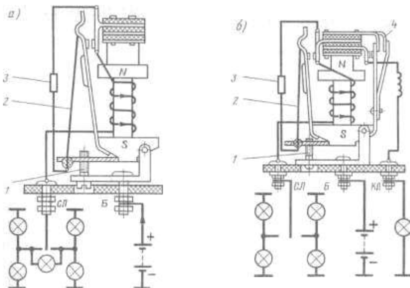
Рис 107 Проверка прерывателей тока указателей поворотов PC57B; PC57 -1-контакты; 2-струна; 3-резистор; 4-планка
