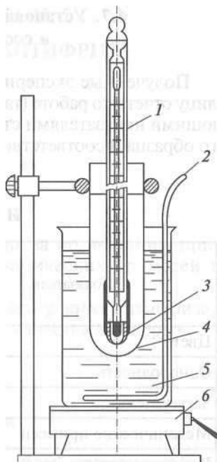
Рис. 12. Прибор для определения температуры каплепадения смазок: 1 — термометр с гильзой; 2-мешалка; 2 — капсуль для испытуемой смазки; 4-пробирка-муфта; 5 — стакан с водой или глицерином; 6—электроплитка
