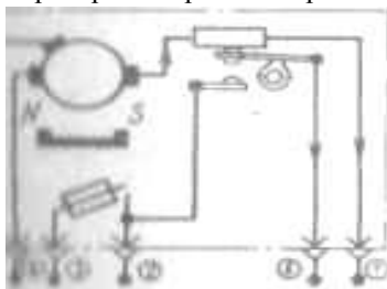
Рис 118 Проверка стеклоочистителя СЛ136: 1 — включение I скорости; 2 — включение II скорости
