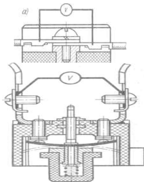
Рис. 128. Проверка падения напряжения: а—на клеммах; б — на зажимах термобиметаллического предохранителя
