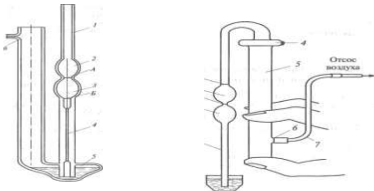
Рис. 11 Заполнение дизельным топливом вискозиметра Пинквейча 1 — узкое колено; 2, 3, 4 — расширительные емкости; 5 — широкое колено; 6 — полый отросток; 7 — резиновая трубка; А, Б — метки
