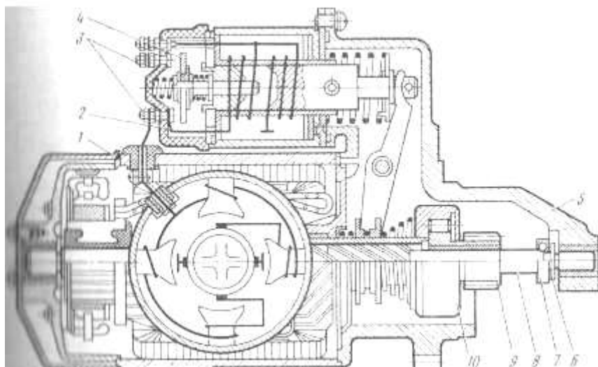
Рис 78 Стартер СТ 230
