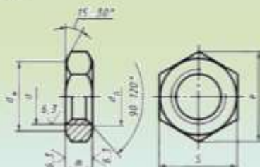
Рисунок 2. Таблица ГОСТ 5916-70
