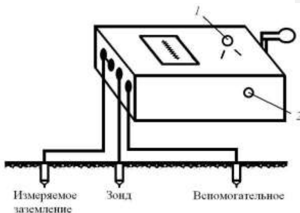
Рис. 9.6. Схема подключения прибора MC08: 1 – переключатель; 2 – реостат
