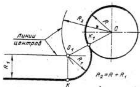
Рис.20 Сопряжение дуги окружности и прямой
