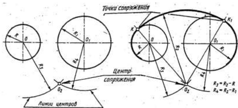
Рис.19 Внутреннее касание
