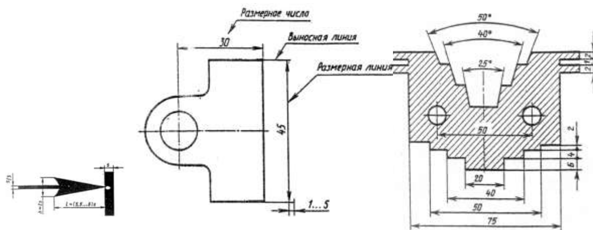
Рис.3 Нанесение размеров
