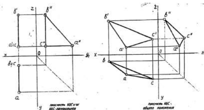
Рис.6 Проекция плоскости
