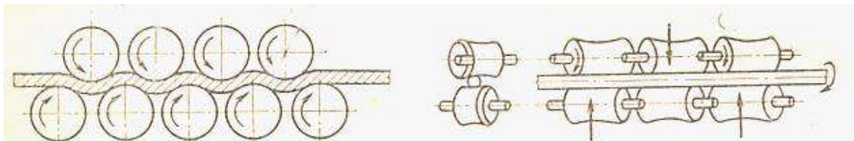
Рис. 1 Окалиноломатель
