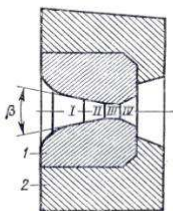
Рис.2. Схема волоки:
